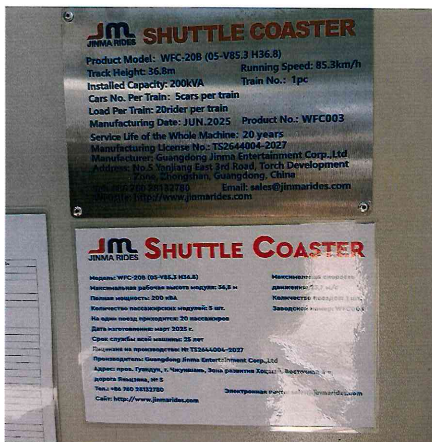
Рисунок 2 – Маркировочная табличка
