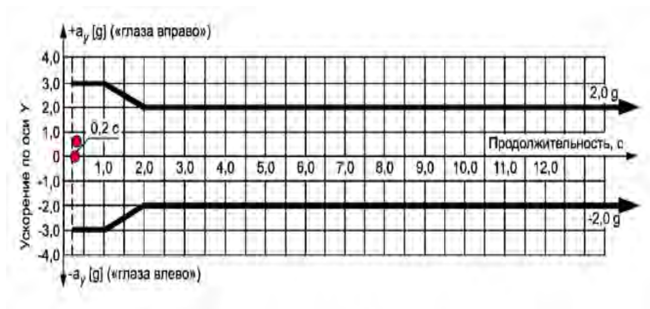
Рисунок А.3 - Пределы по времени для допустимых ускорений в направлении Y
